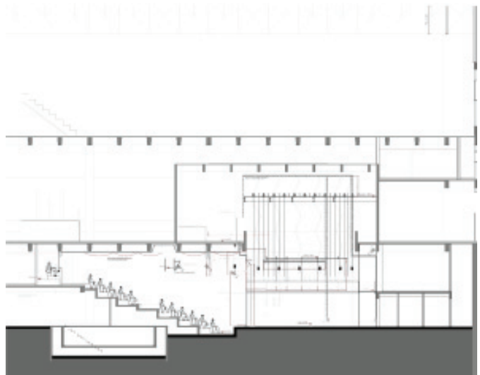
Figuras 20 e 21: Planta do teatro e corte geral. Sesc Santana, 2000 Fonte: Daniela Zilio, a partir do projeto de autoria de José Carlos Serroni e Gustavo S. Lanfranchi
